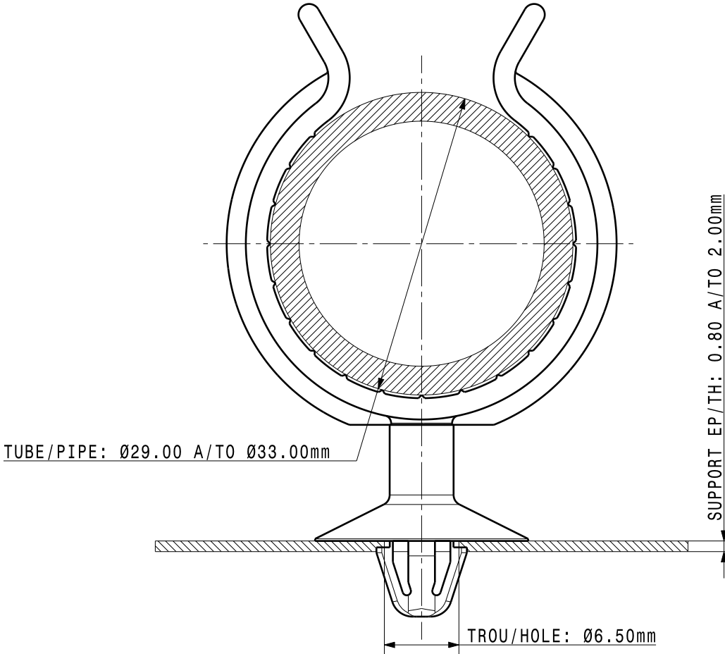
EXEMPLE D'UTILISATION / USE CONDITION ECHELLE / SCALE: 2:1
