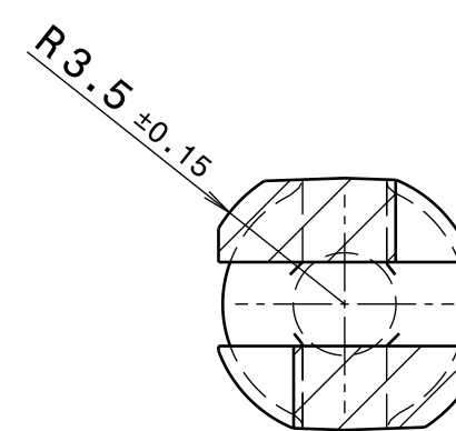
Schnitt / Section B-B
