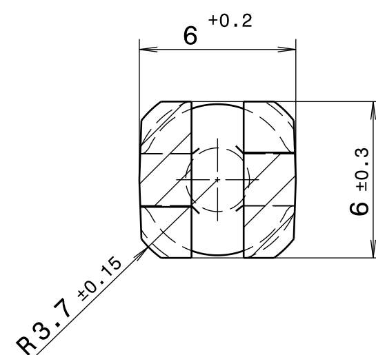
Schnitt / Section A-A
