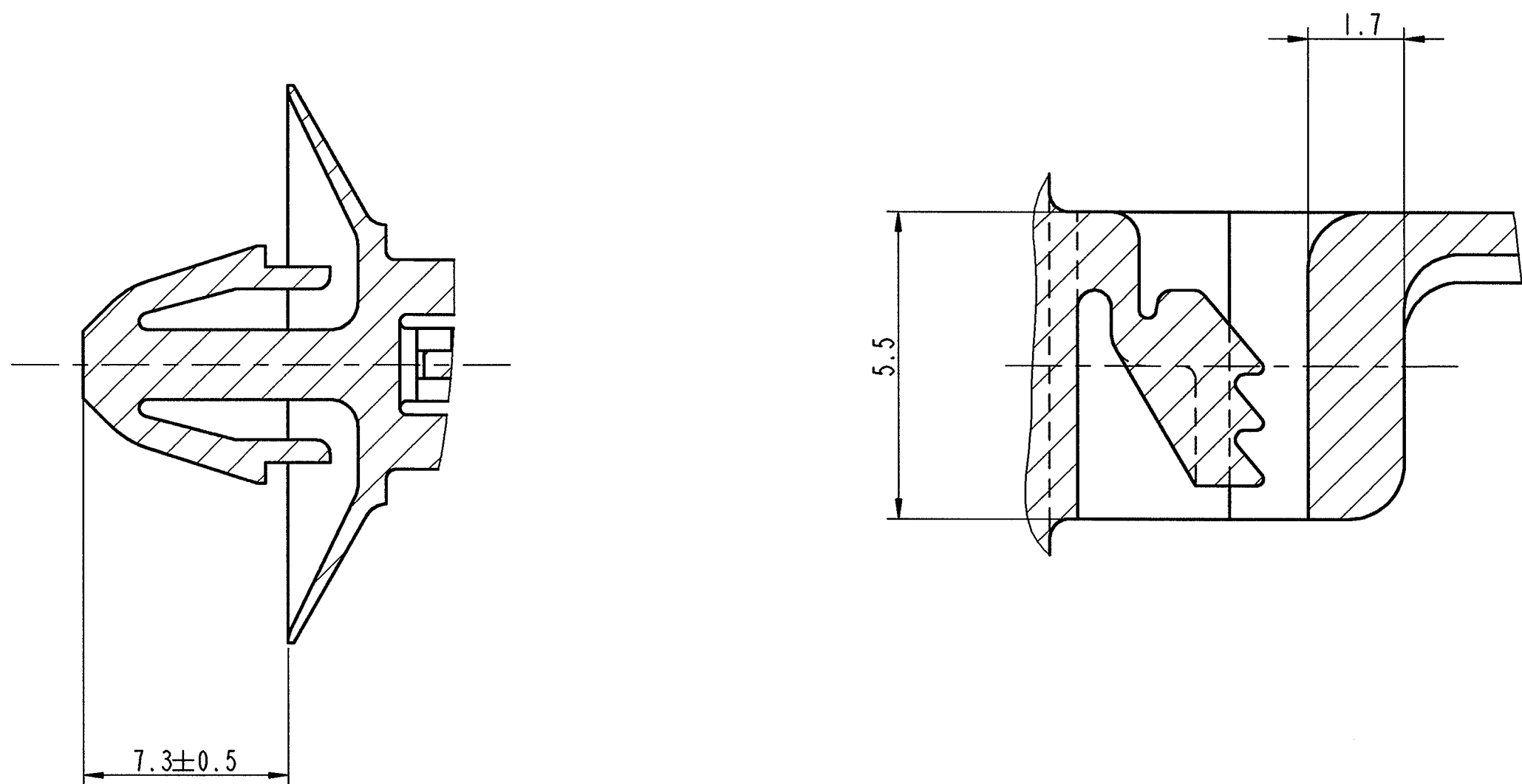
Einzelheit/detail Z 10:1
