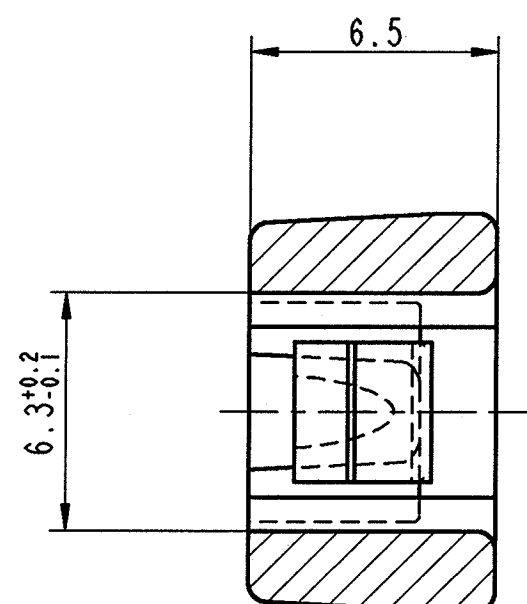
Schnitt/section A-A
