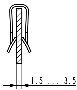
Einbausituation / assembly situation 2:1
