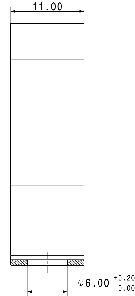
COUPE A-A / CUT A-A
